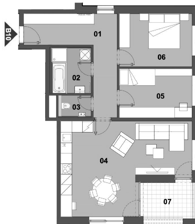
SCHÉMA PODLAŽÍ
