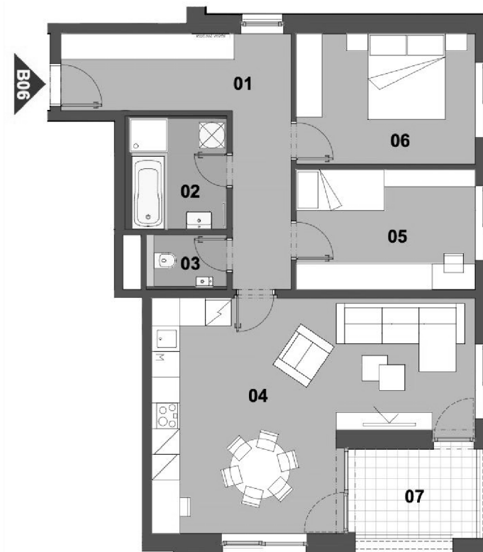
SCHÉMA PODLAŽÍ
