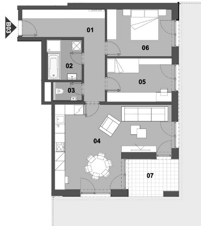
SCHÉMA PODLAŽÍ
