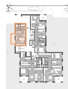
SCHÉMA PODLAŽÍ
