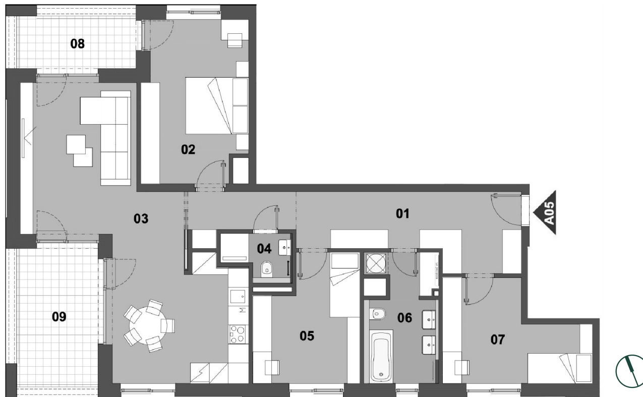
SCHÉMA PODLAŽÍ
