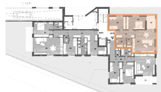
SCHÉMA PODLAŽÍ
