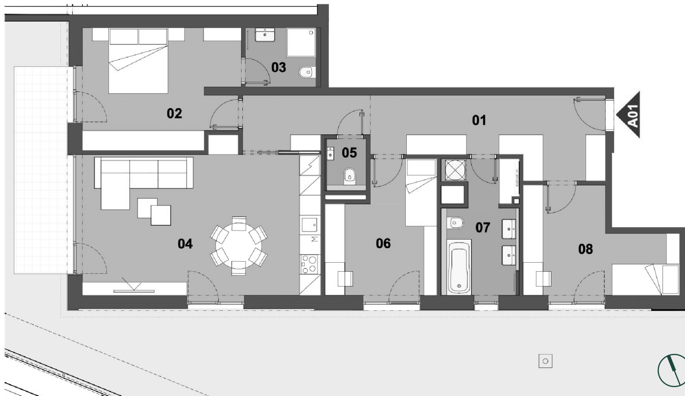
SCHÉMA PODLAŽÍ
